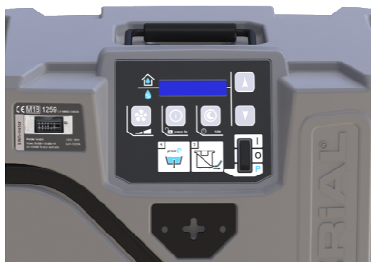
Bedientableau
