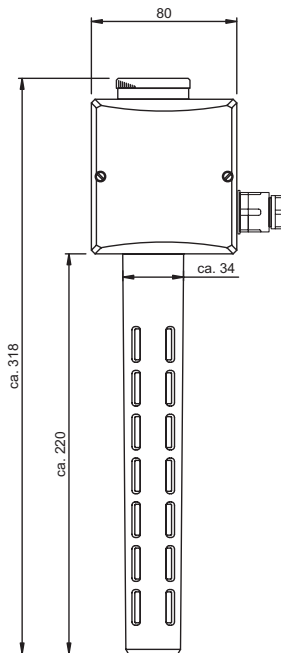
Hygrostat Frontansicht
